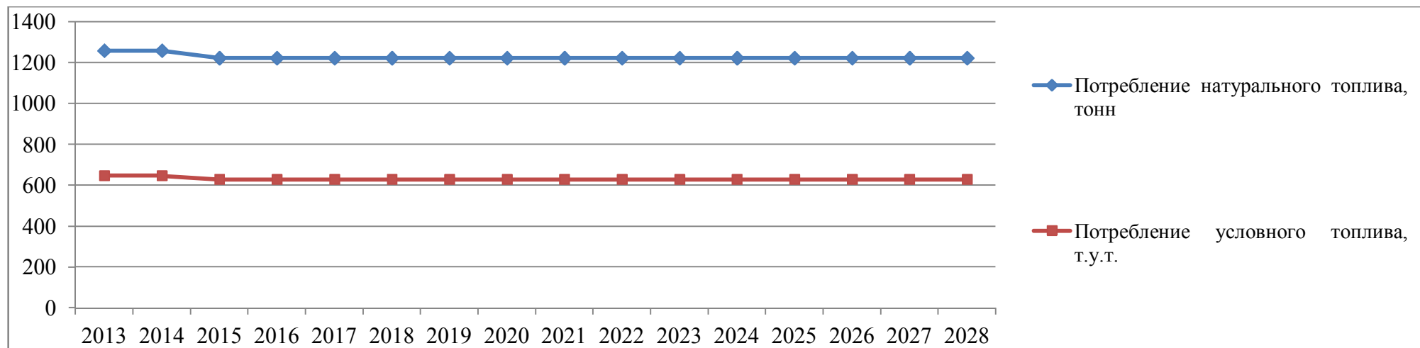
Рисунок 8.1. Перспективный топливный баланс котельной п. Ойский
